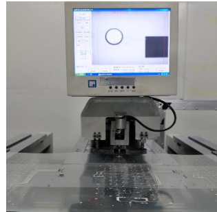
沖定位孔
